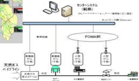
②ガバナ遠隔監視システム
