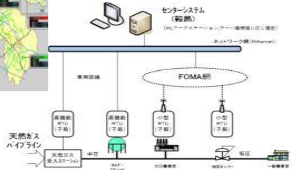
②ガバナ遠隔監視システム
